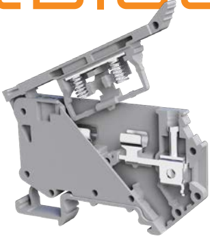
FDT 4 L
