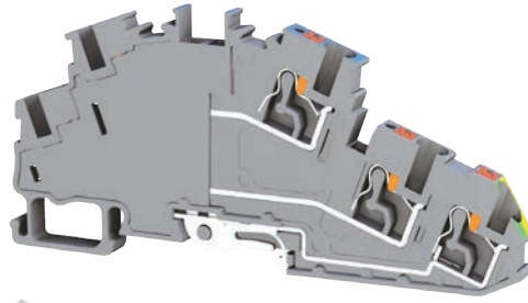
PFT 2,5 2P+E (Linye Klemensi)
