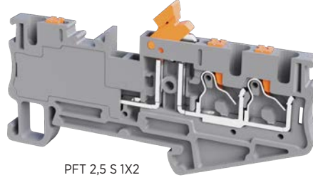
PFT 2,5 S 1x2
