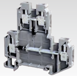
8002099298 TBL 4 2P X4
